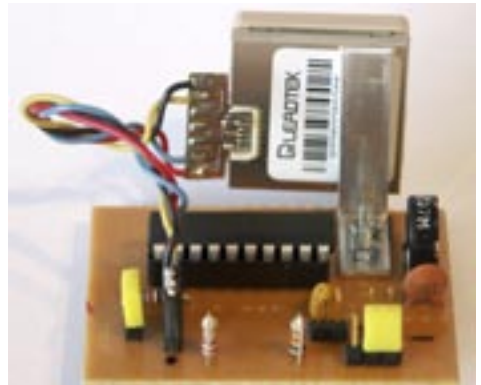
Platine mit GPS-Modul
